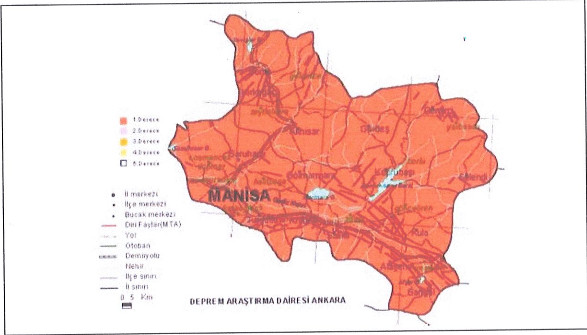
Manisa İli Diri Fay Hatları
